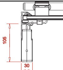
Montage Perpendiculaire au rideau (B)
