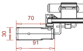
Montage Parallèle au rideau (A)
