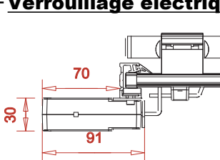
Montage Parallèle au rideau (A)
