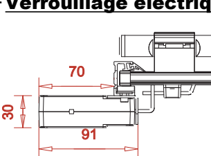
Montage Parallèle au rideau
